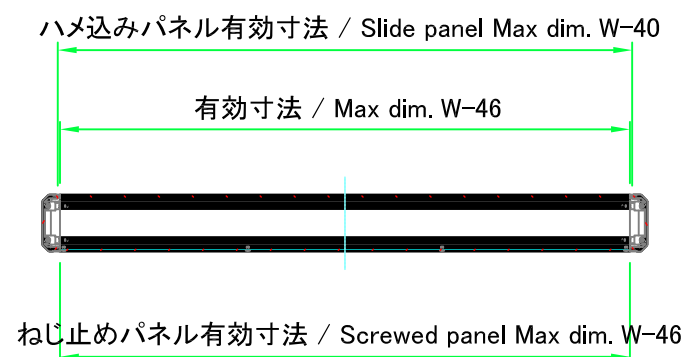
A-A ( 1 : 10 )
