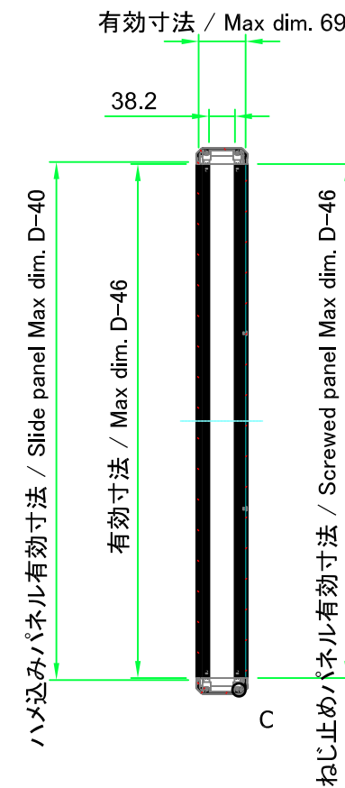
B-B ( 1 : 10 )
